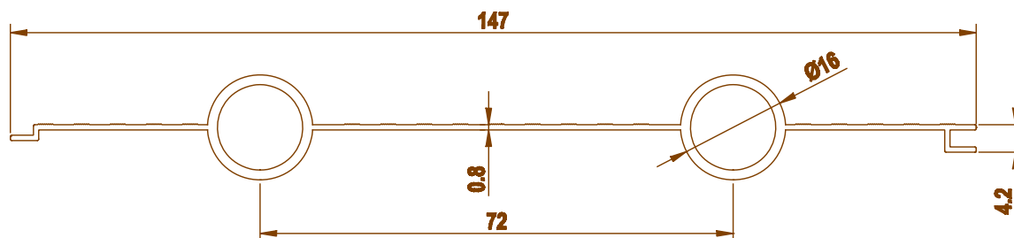
2595 0.648 kg/m
