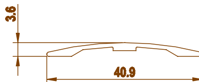
3710 0.180 kg/m
