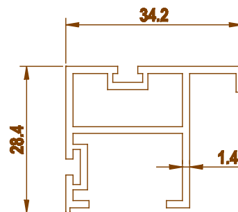
3708 0.502 kg/m
