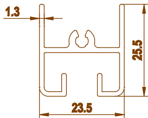
3535 0.375 kg/m
