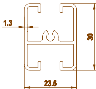
3536 0.453 kg/m
