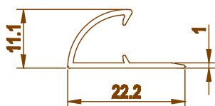
3253 0.110 kg/m
